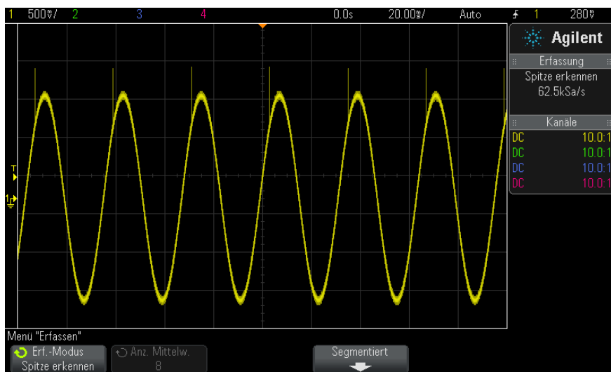
Abbildung 37 Sinus mit Störimpuls, Modus „Spitze erkennen“
