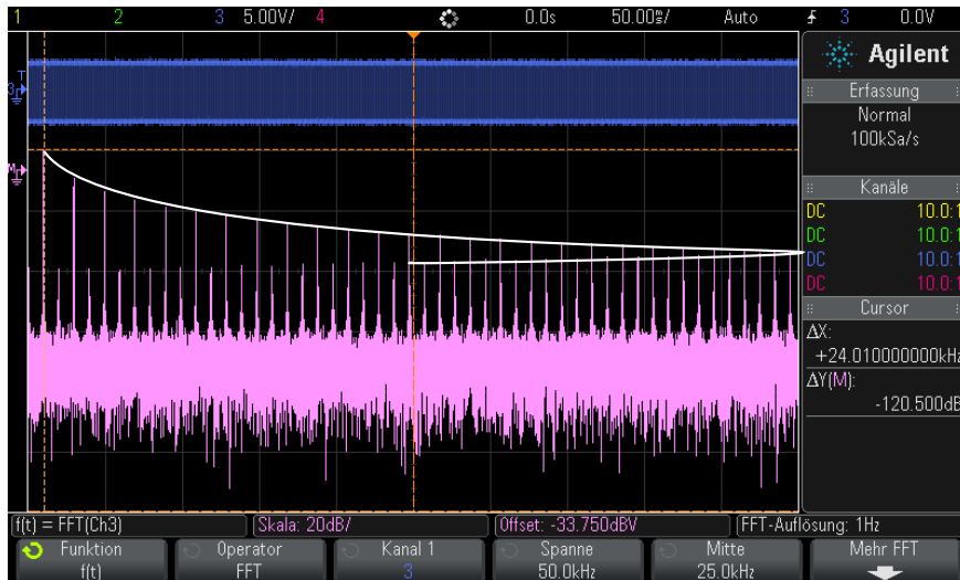
Abbildung 9 Aliasing
