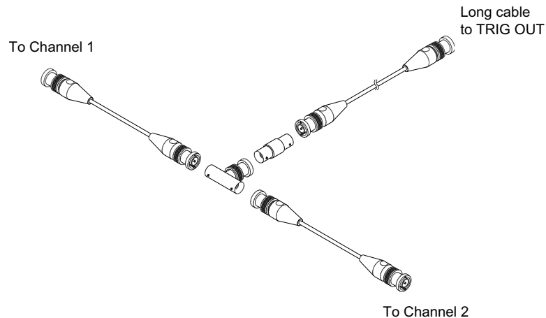
Abbildung 48 Kabel für die benutzerdefinierte Kalibrierung für 2-Kanal-Oszilloskop
