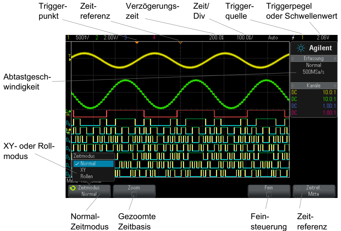
Abbildung 2 Menü „Horizontal“
